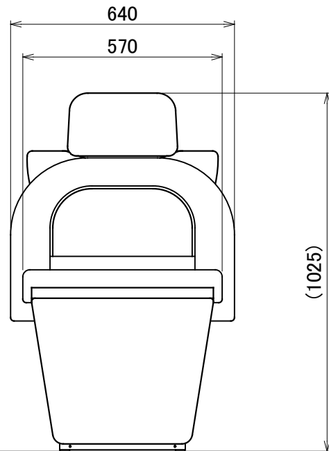
ベースマウント図(A 矢視)
