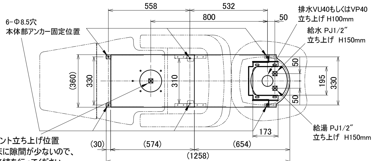
ベースマウント図(A 矢視)
