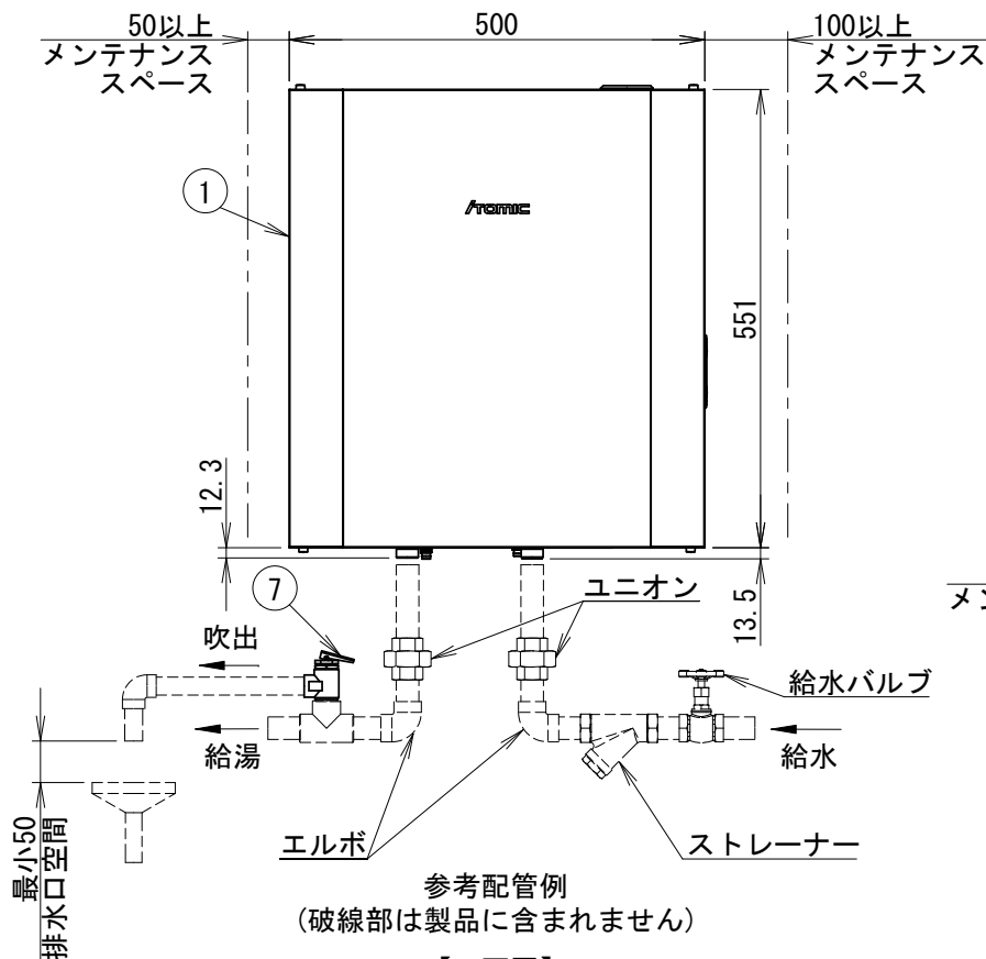
【正面図】
