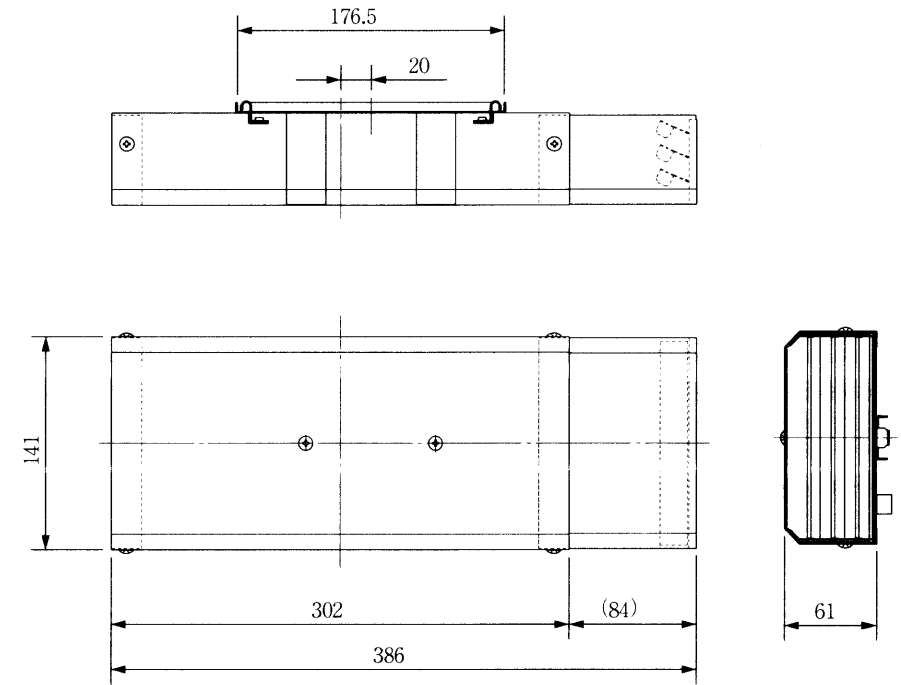
側方排気アダプタ寸法図 (S=1/5)
