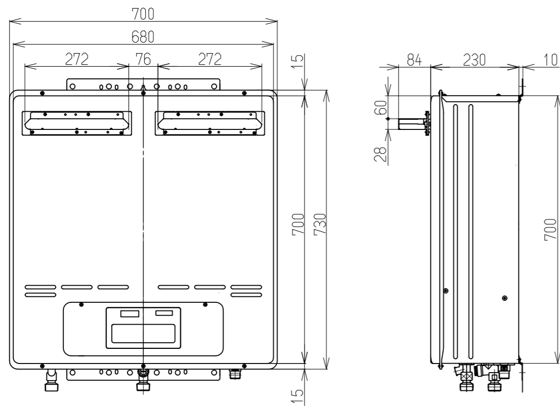
排気カバー取付図
