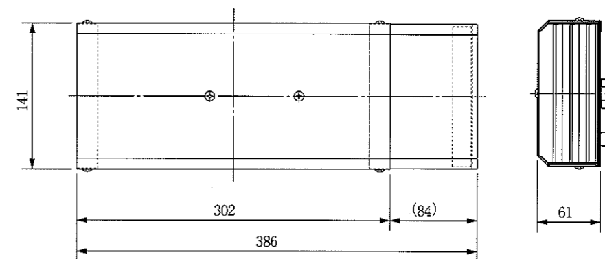
側方排気アダプタ寸法図 (S=1/5)
