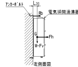
左側面図 計算モデル図
