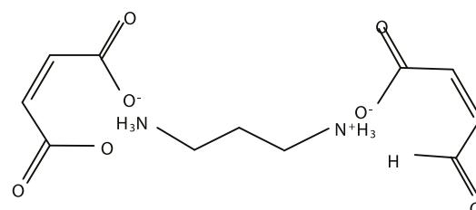
ジマレイン酸プロピレンジアンモニウム
