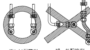
正しい配管例
