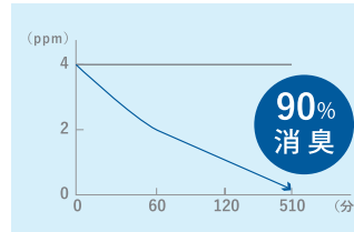
硫化水素
