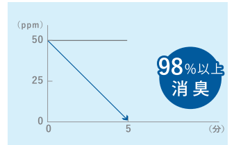
酢酸
